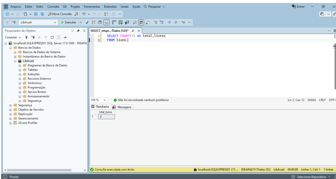
Figura 11 - Livros SQL.
