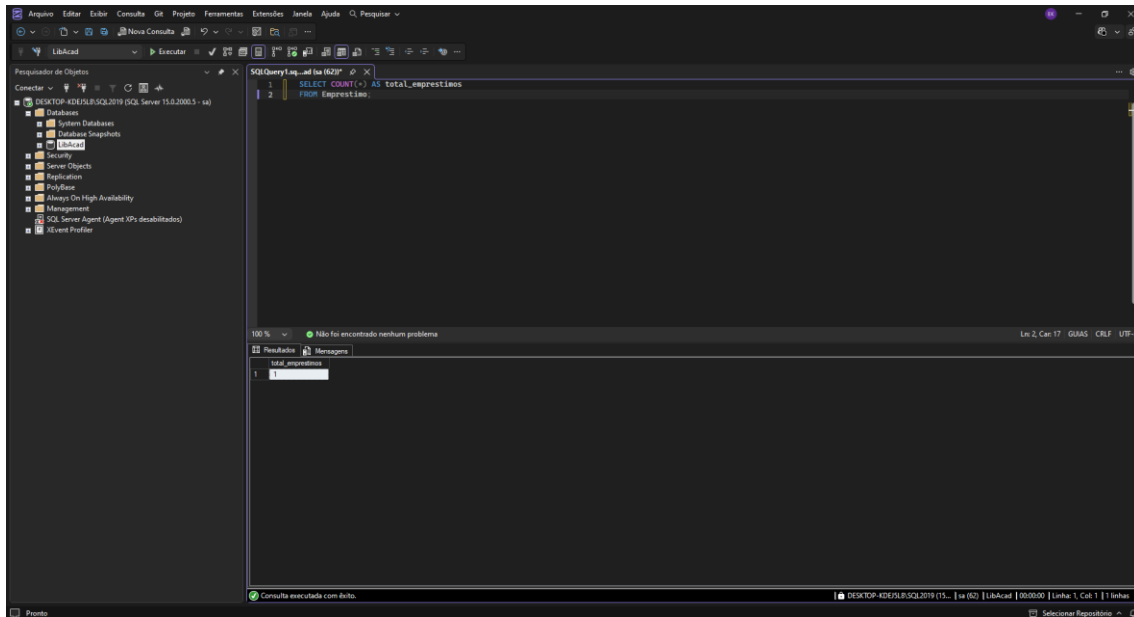
Figura 13 - Empréstimo SQL.
