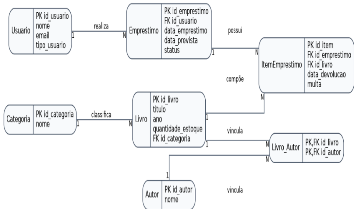
Figura 1 - Diagrama ER
