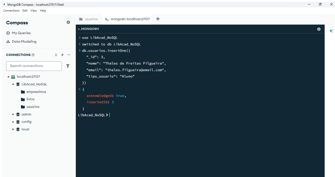
Figura 22 - Criando usuário.
